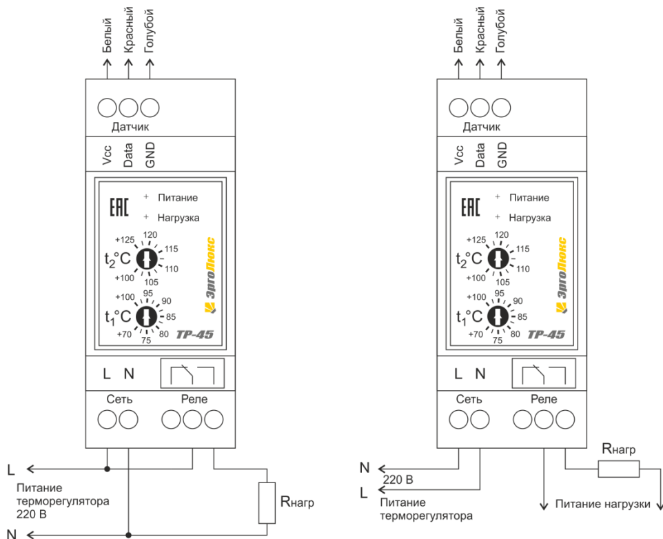
Схема 1. Подключение терморегулятора и нагрузки к общей сети питания
