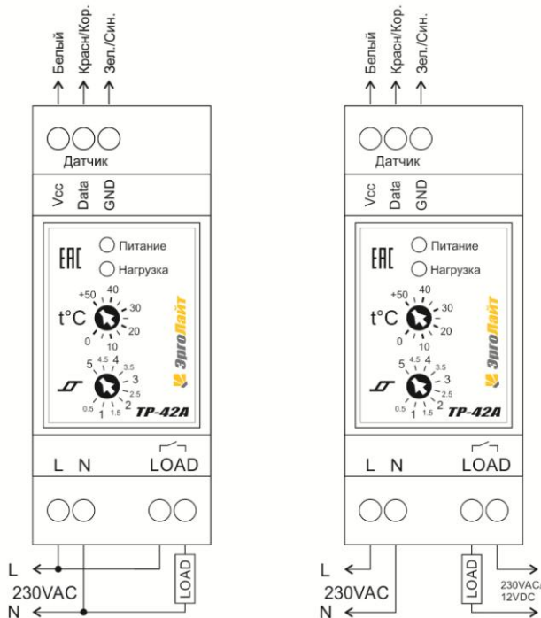
Схема 1. Подключение терморегулятора и нагрузки к общей сети питания
